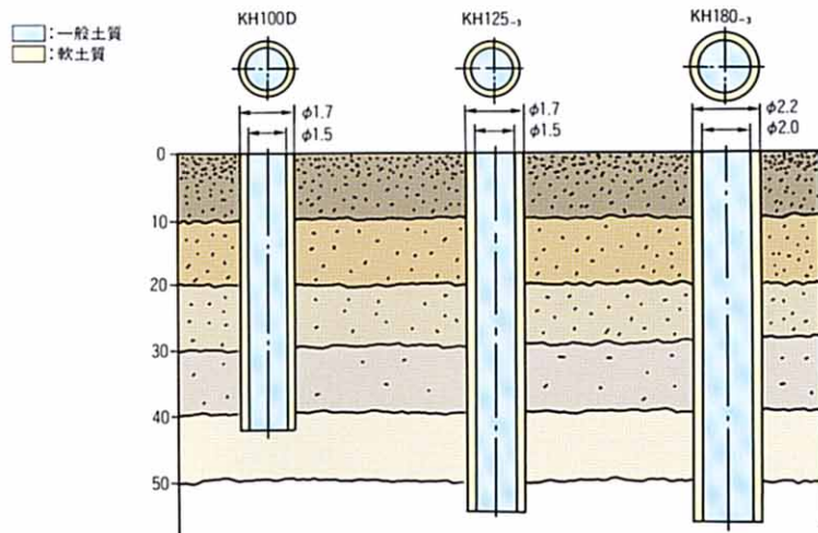
日立アースドリル掘削径および掘削深度比較
